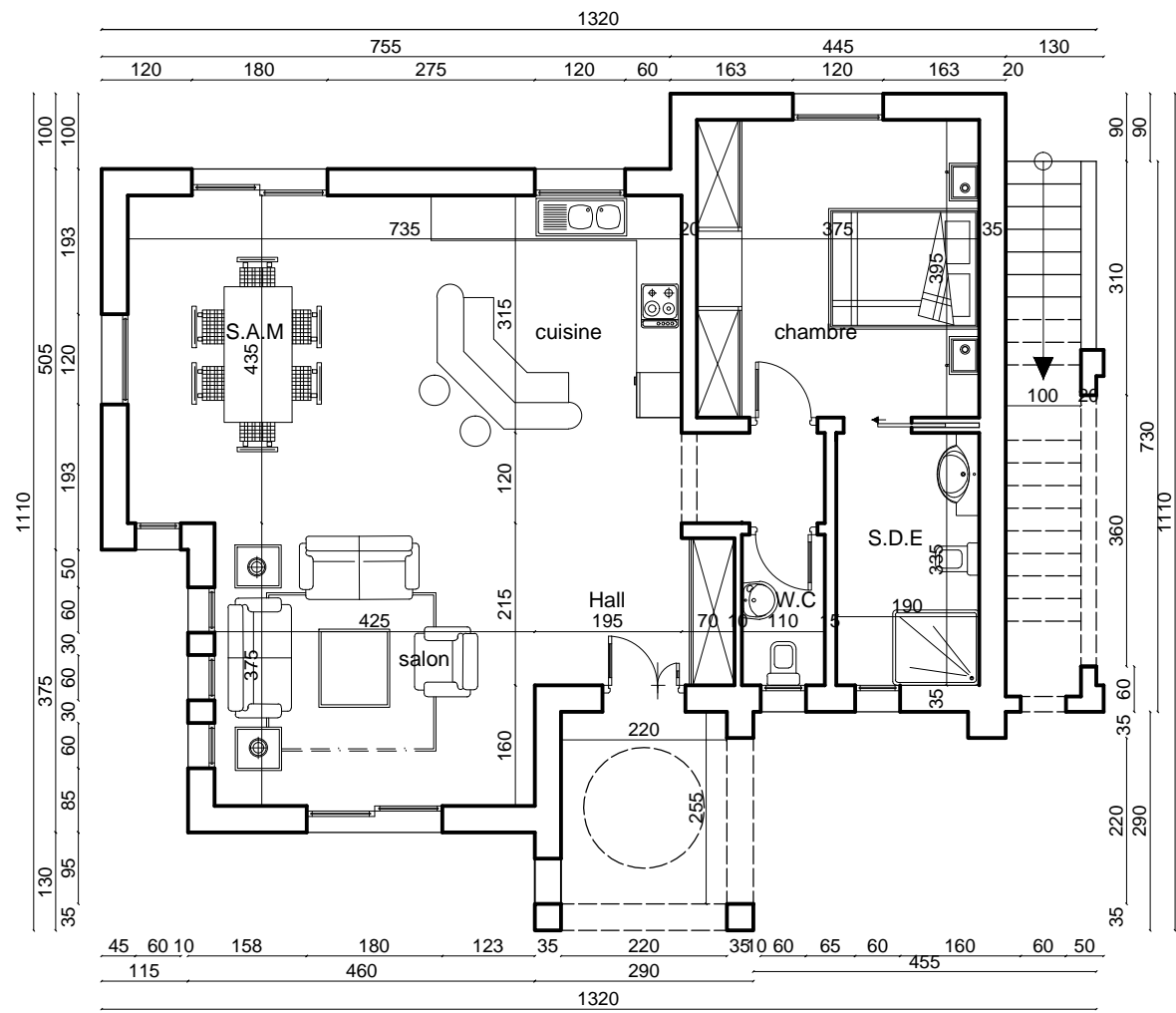
Plan RDC sc: 104m 2 sc esc: 8.7m 2
