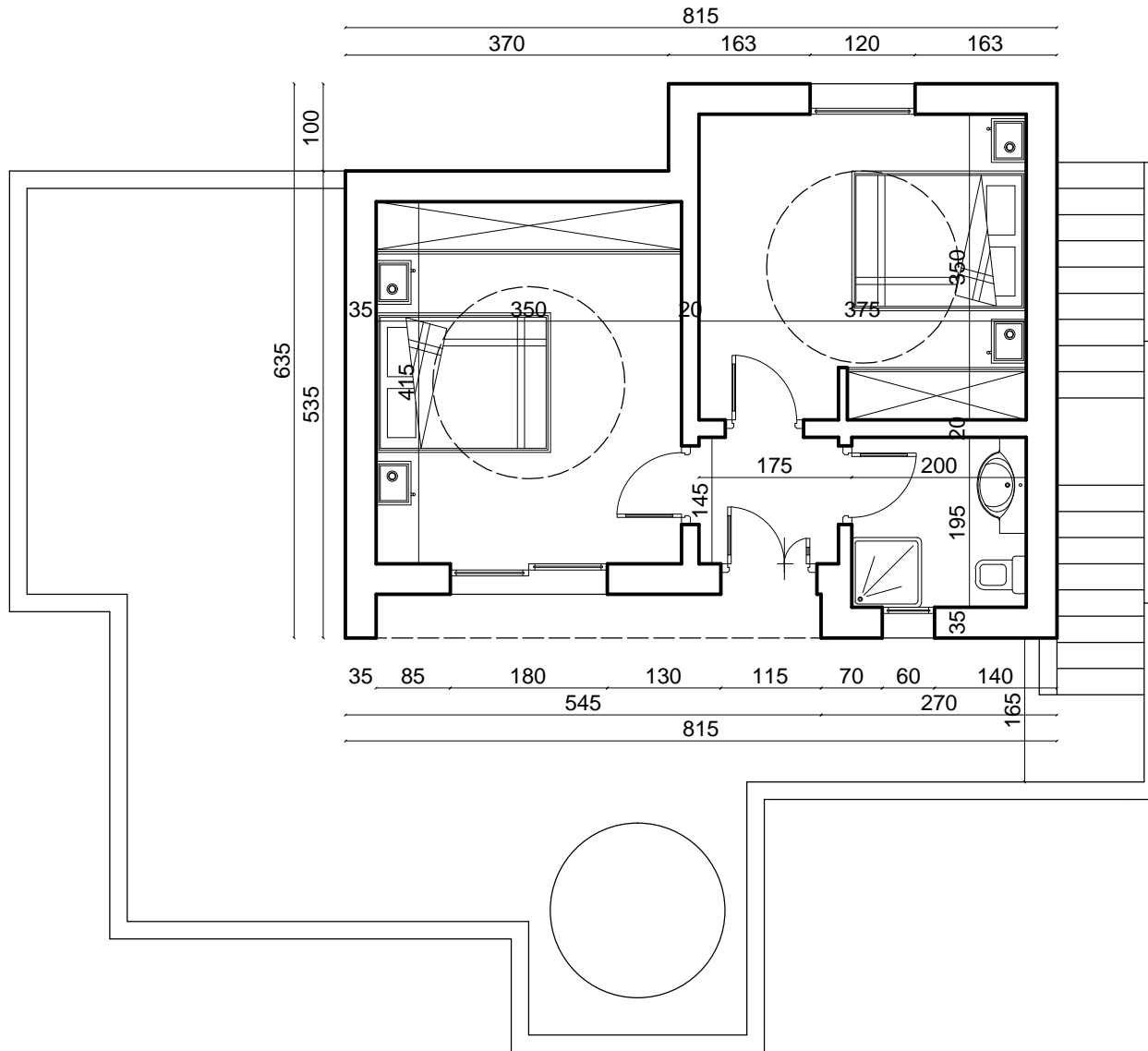
Plan RDC sc: 48m 2
